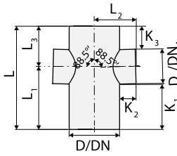
Derivación doble 88° 30'
